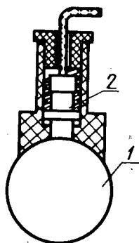
1 — объект контроля; 2 — преобразователь вихретокового измерителя
